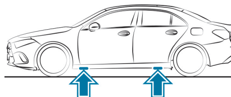
Расположение опорных точек для подъема домкратом
