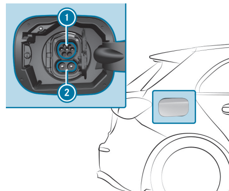
Розетка автомобиля, тип Combo 2 (пример)
