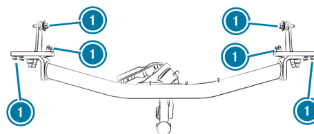
Точки крепления (не подключаемый гибрид)
