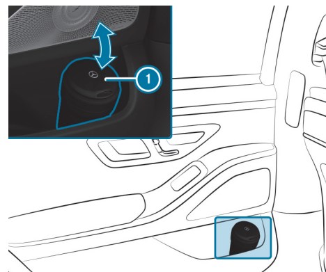
Пепельница в задней двери (пример)
