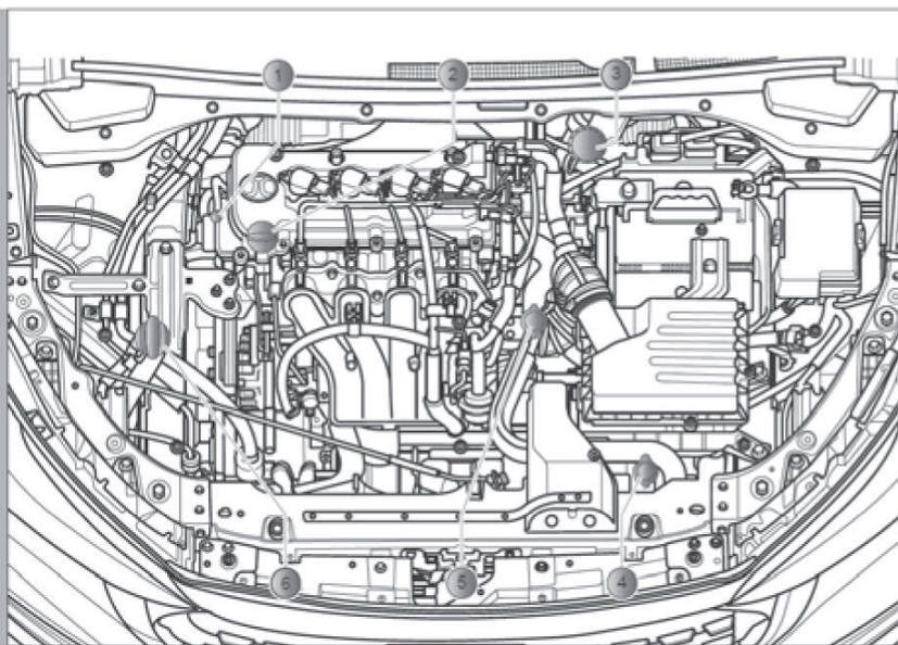
Компоновка моторного отсека (Модель A151A1)
