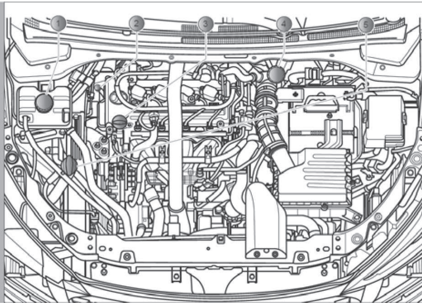
Компоновка моторного отсека (Модель A151R1)
