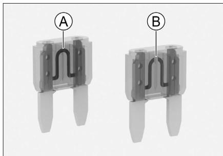
А Исправный предохранитель
